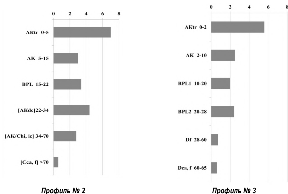
Рис. 2. Содержание гумуса в криоаридных выщелоченных вытоптаных почвах, %
